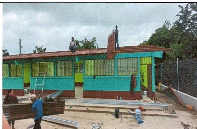
Foto 4: Mejoramiento de la cubierta metálica del Instituto (techo), con lámina troquelada No. 24 con canal para agua pluvial y bajantes fabricados en tuvos PVC.
